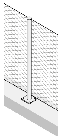
A | Standard Mittelpfosten Ø 42,4 mm
