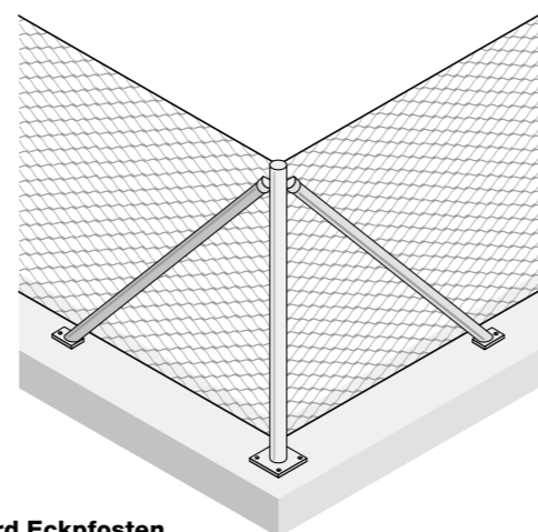
B | Standard Eckpfosten Ø 48,3 mm Komplett mit Reling, zwei Streben und Seilumlenkung.
